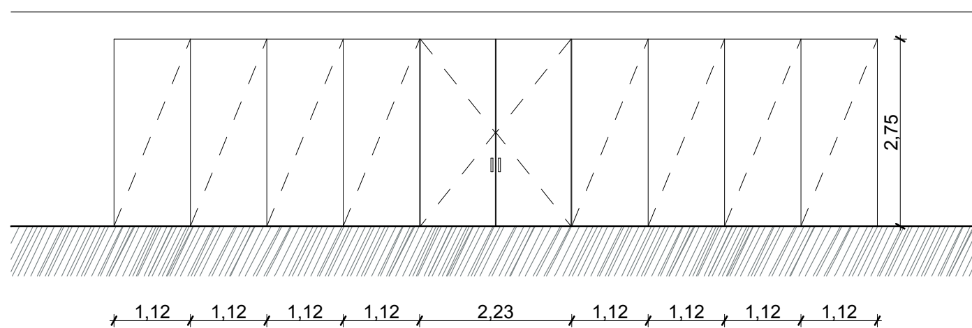
PORTÁL NÉZET
