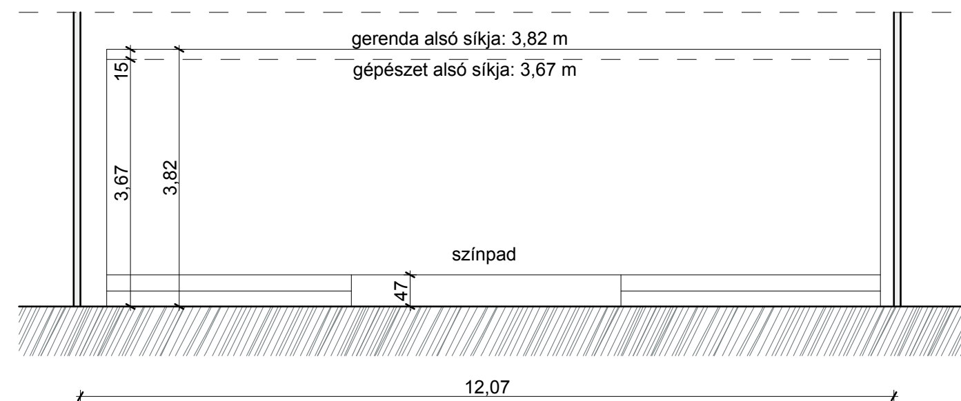
METSZET
